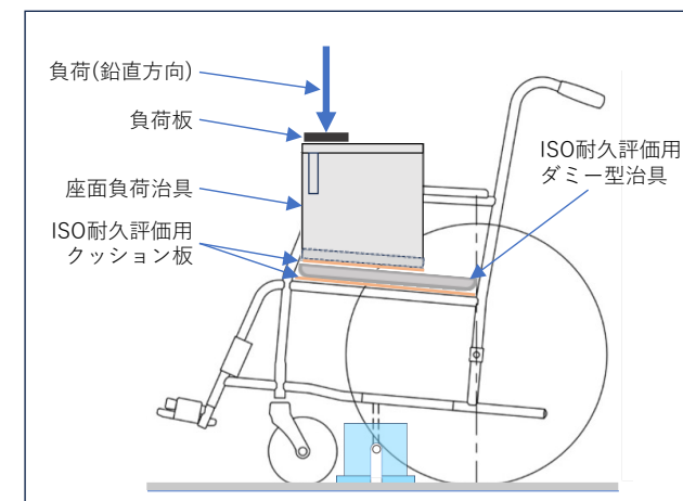
車載車椅子静的試験法(一部)
